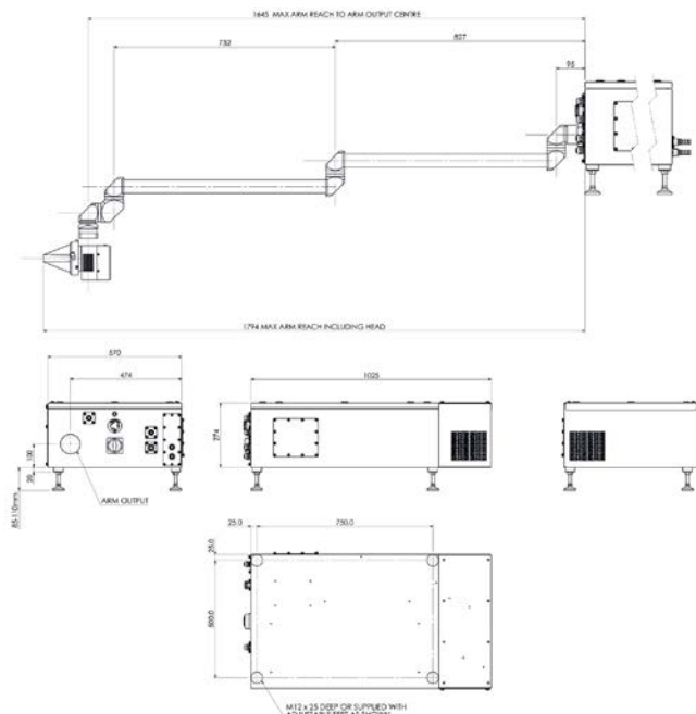
寸法 (mm)
